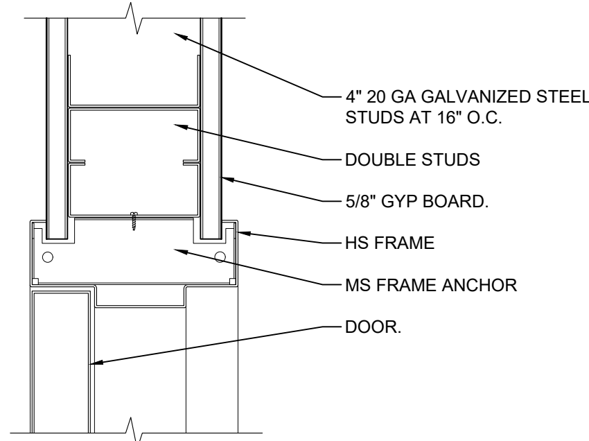
3 DOOR HEAD (JAMB SIM) scale 3"=1'-0"
